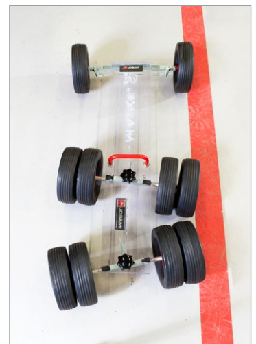
Snedställda och oparallella axlar Out of square and non-parallel axles Schräg und unparallele Achsen
