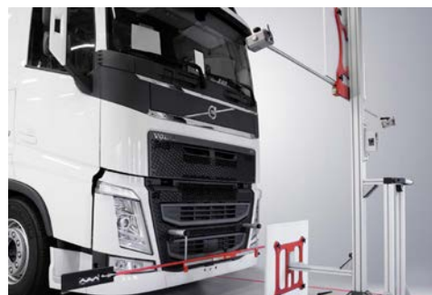
Einstellung von ACC-, FLS/LPOS- und LDWS-/MFC-Systemen
