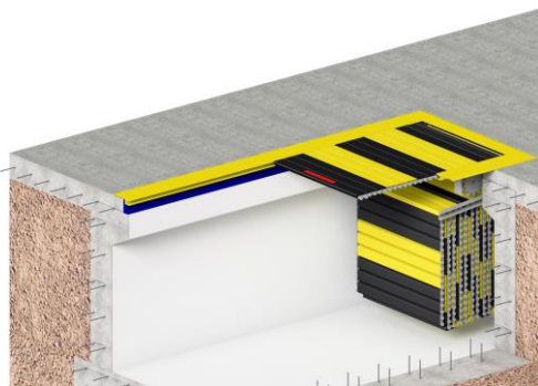
Querschnitt einer ASP Grubenabdeckung
